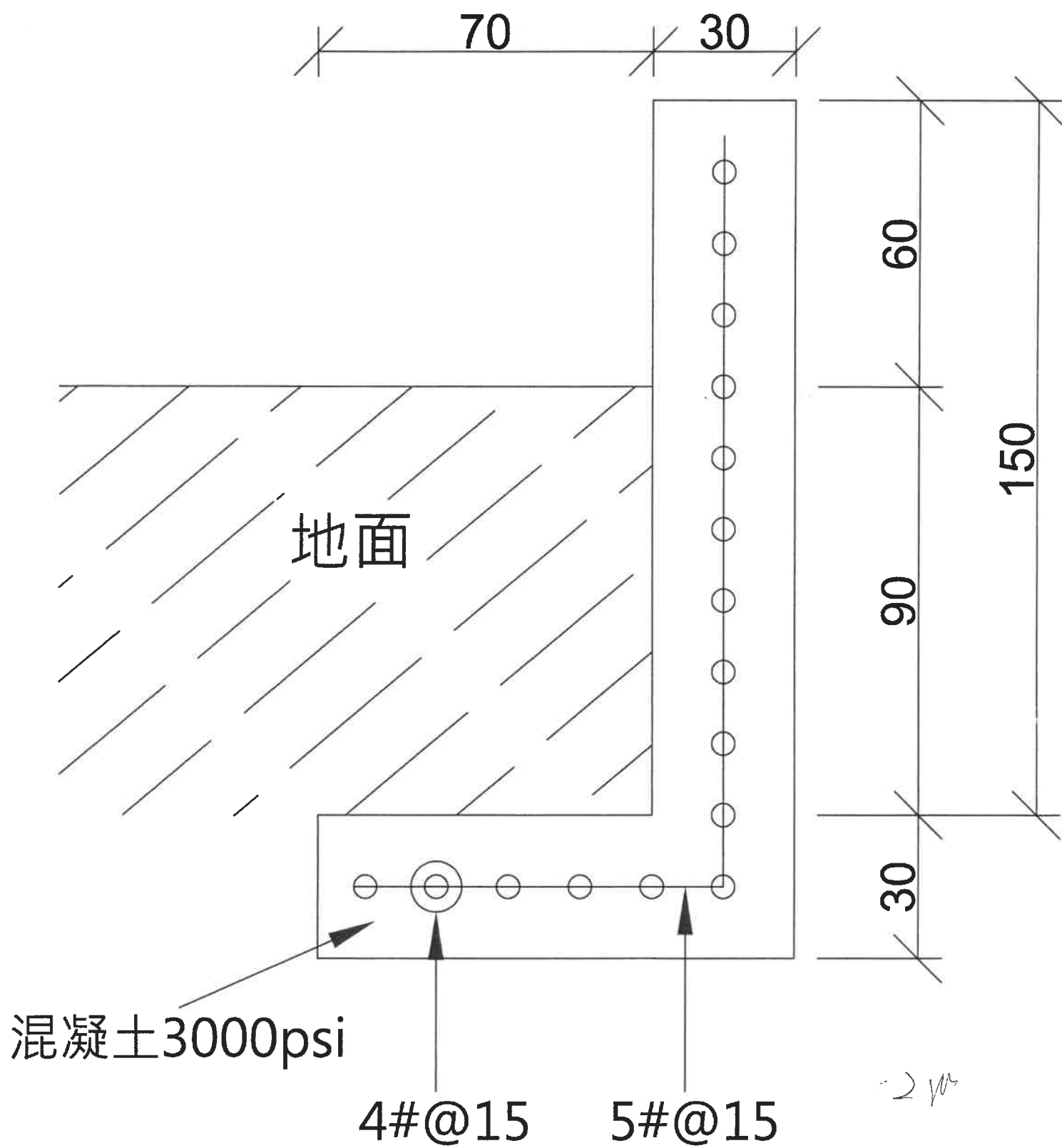
L型擋土牆
